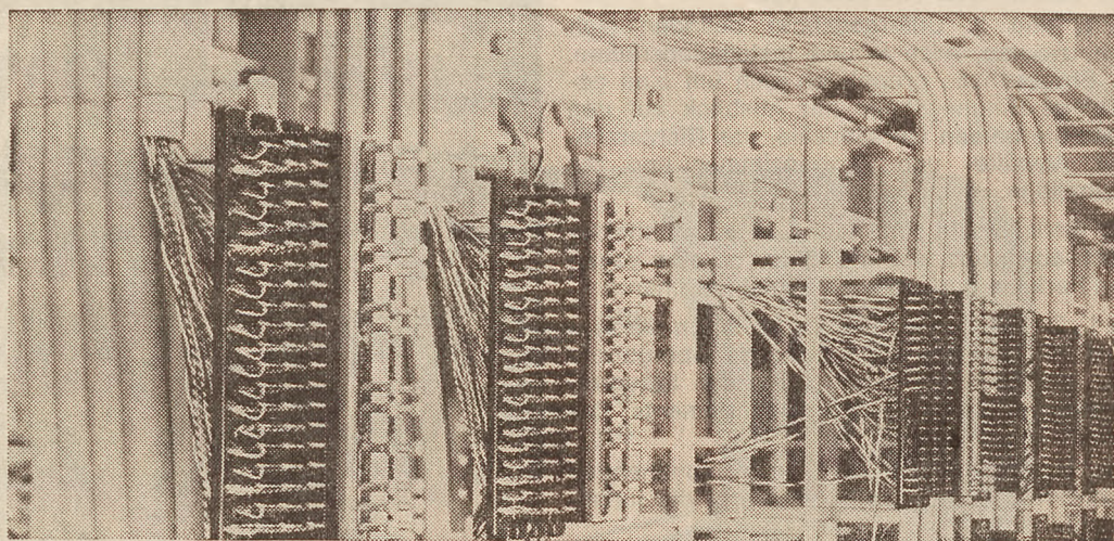
Telephonkabel für automa- tische Zentralen
